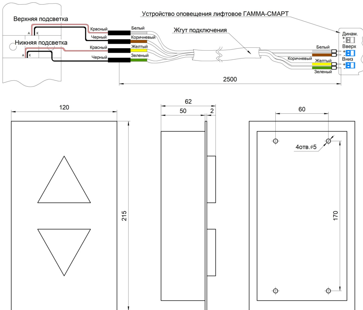
Рис.1 Внешний вид «Указатель лифтовой» НШЕК.468232.209
